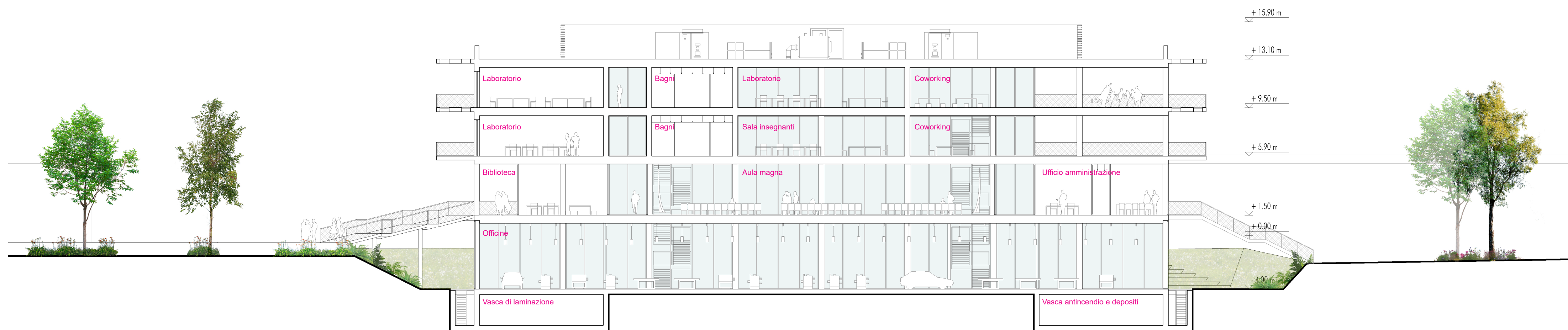
Sezione BB | 1:200
