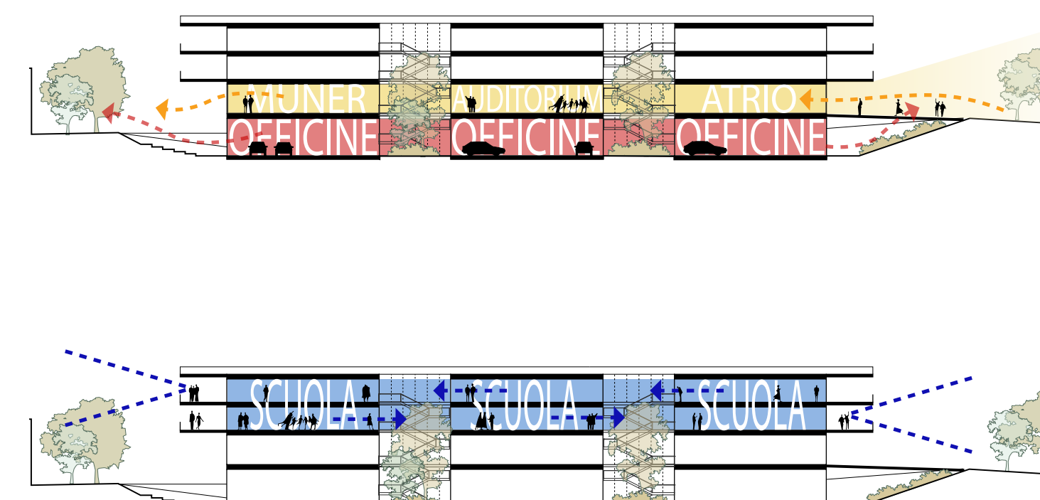
Sezioni funzionali
