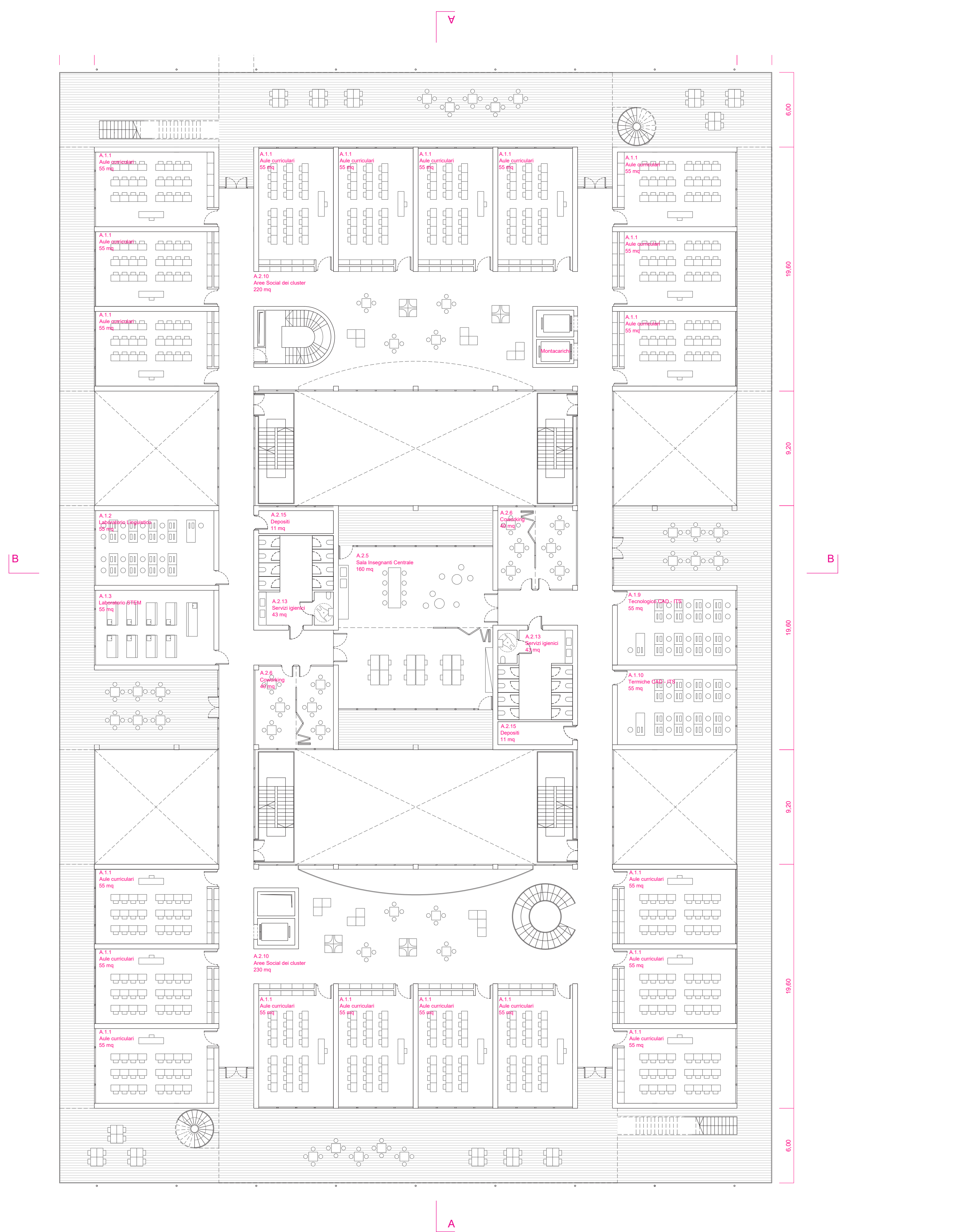
Pianta piano 1 | 1:200
