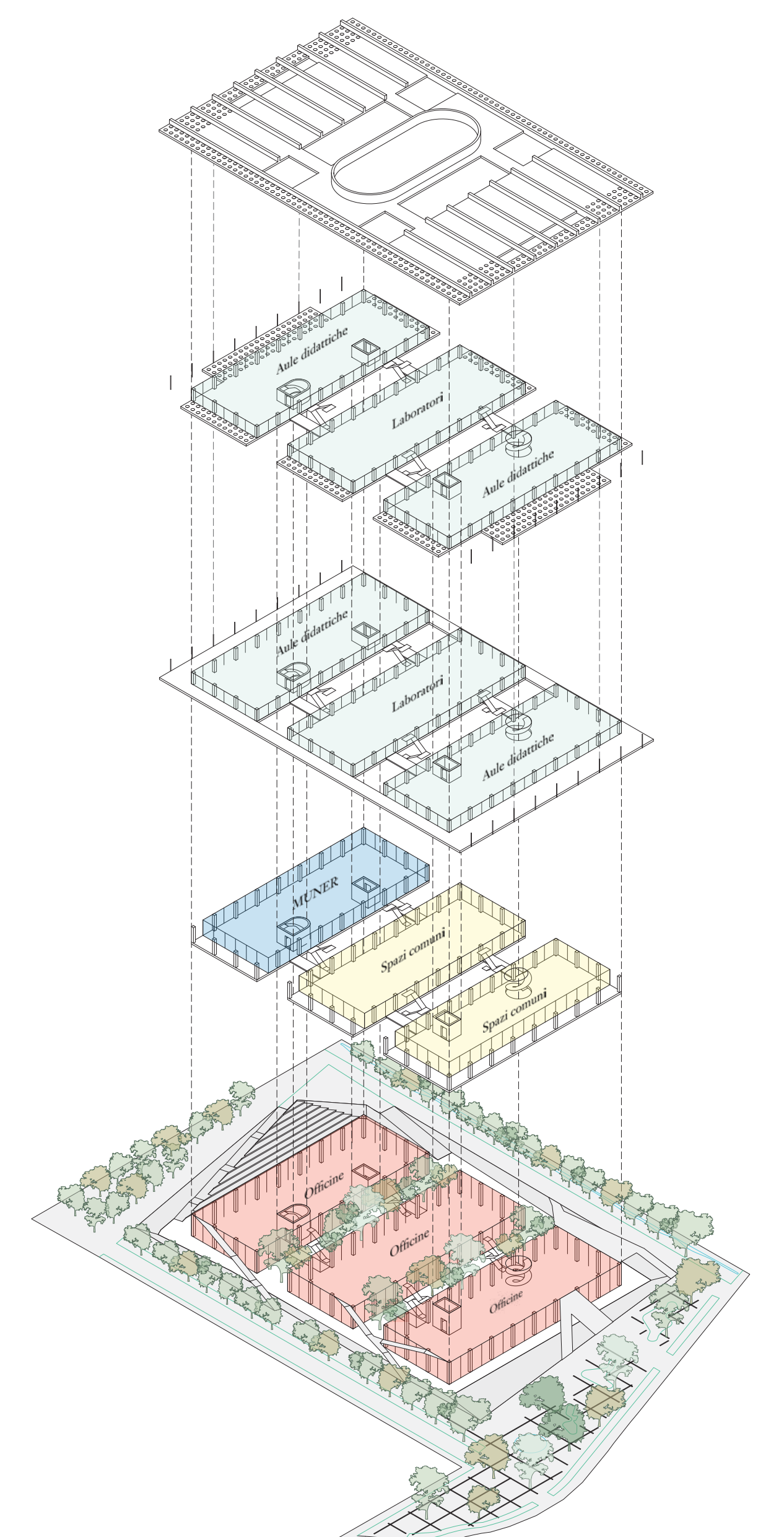
Esplso funzionale
