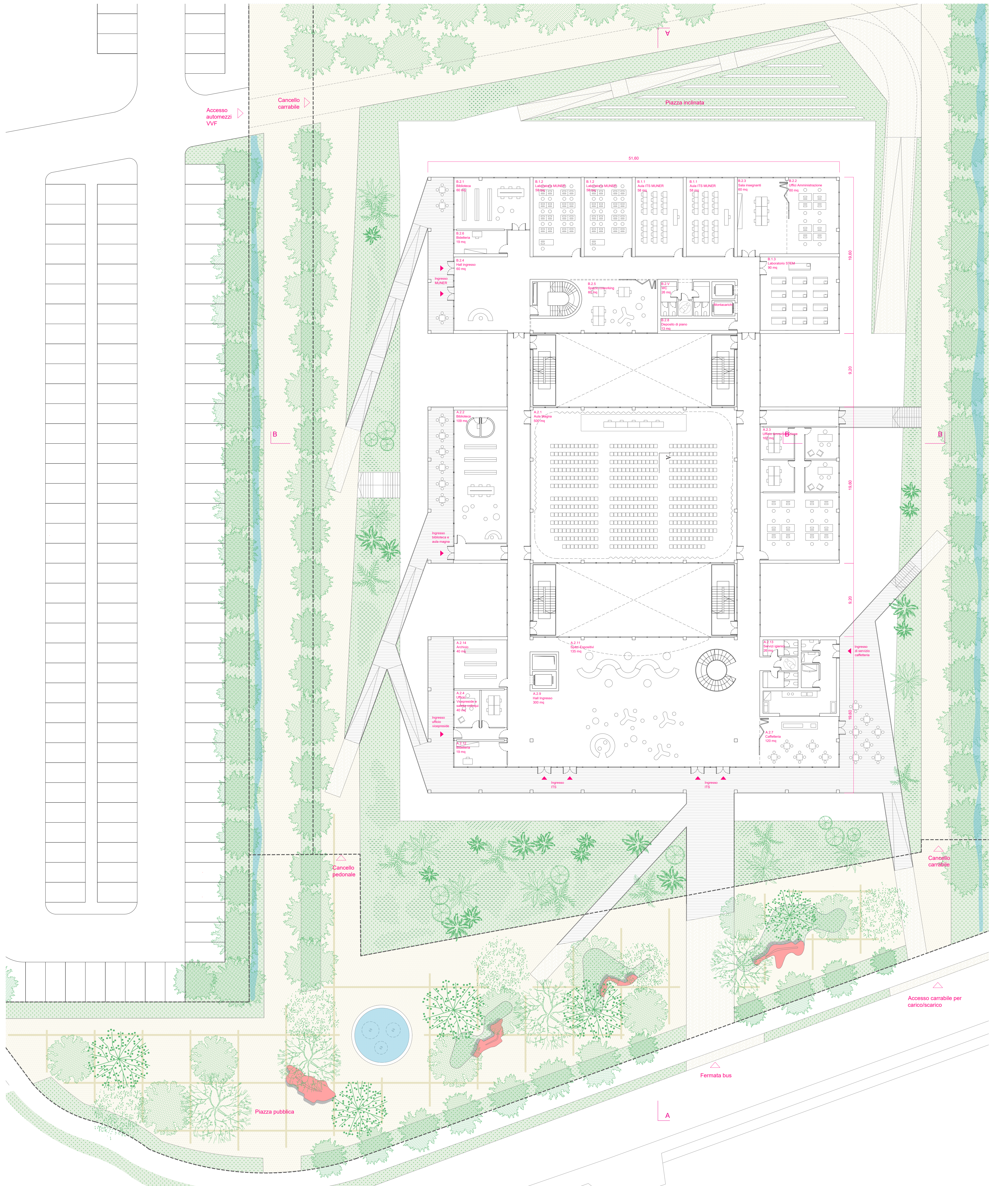
Pianta piano terra superiore | 1:200
